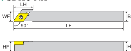
寸法 Dimension(mm)
