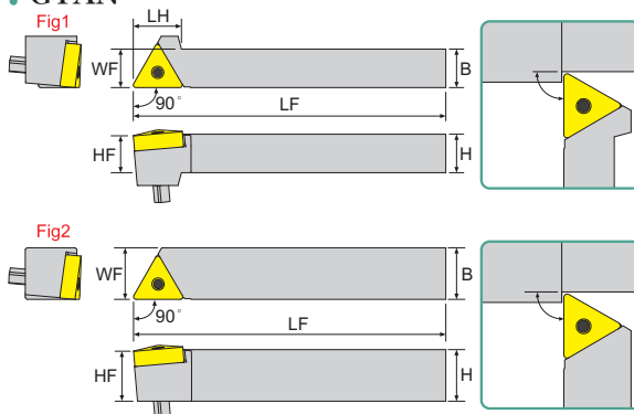
寸法 Dimension(mm)
