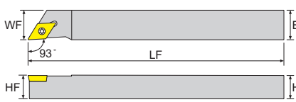
寸法 Dimension(mm)
