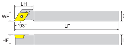
寸法 Dimension(mm)
