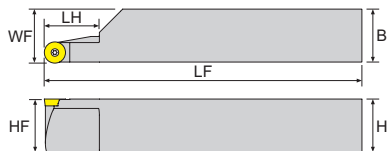
寸法 Dimension(mm)
