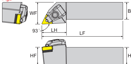
寸法 Dimension(mm)
