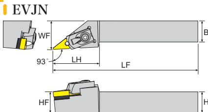
寸法 Dimension(mm)
