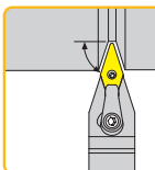
夾持方式 Clamping System
