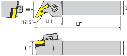
寸法 Dimension(mm)
