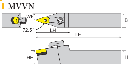
寸法 Dimension(mm)
