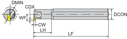
寸法 Dimension(mm)
