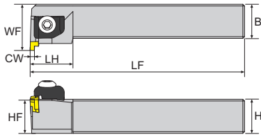
寸法 Dimension(mm)
