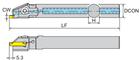
寸法 Dimension(mm)
