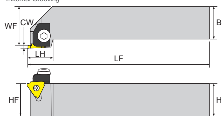
寸法 Dimension(mm)
