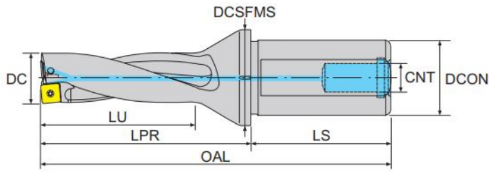
寸法 Dimension(mm)
