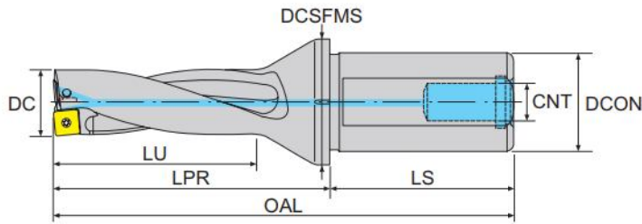
寸法 Dimension(mm)
