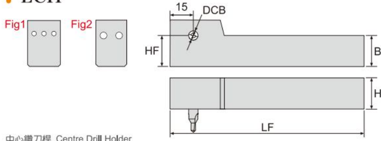
寸法 Dimension(mm)
